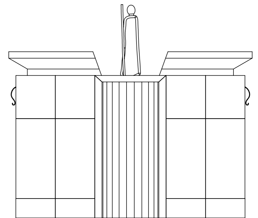
SEZIONE C-C
